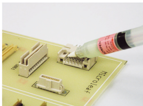
Нанесення флюсу
